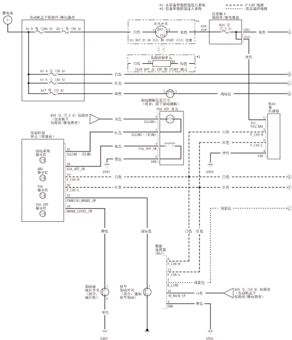
VSA 系统电路图
